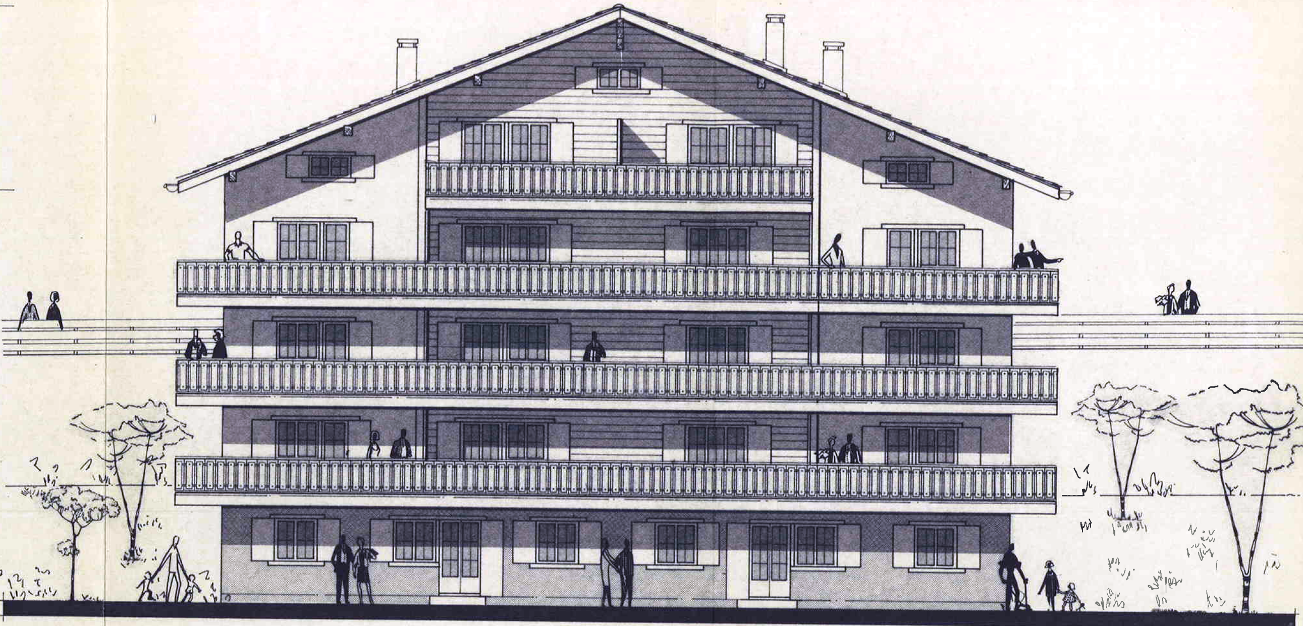
FAÇADE OUEST
